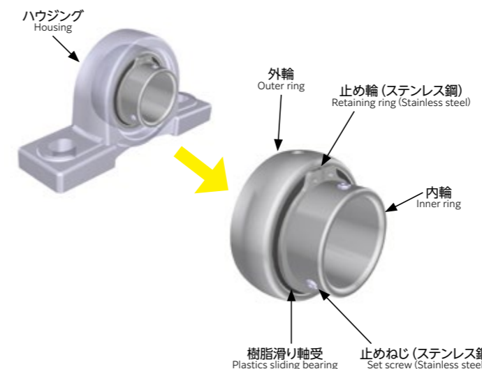
図5-16 樹脂滑りベアリングユニットの構造 Fig.5-16 Structure of plastics sliding bearing unit
