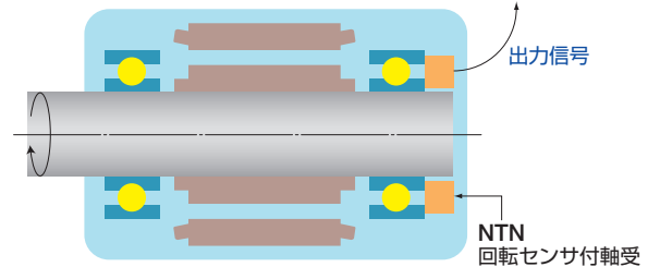
図 モータへの適用例
